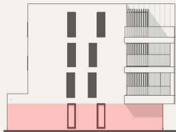
Linkergevel
