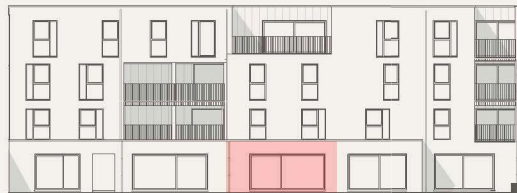
Achtergevel
